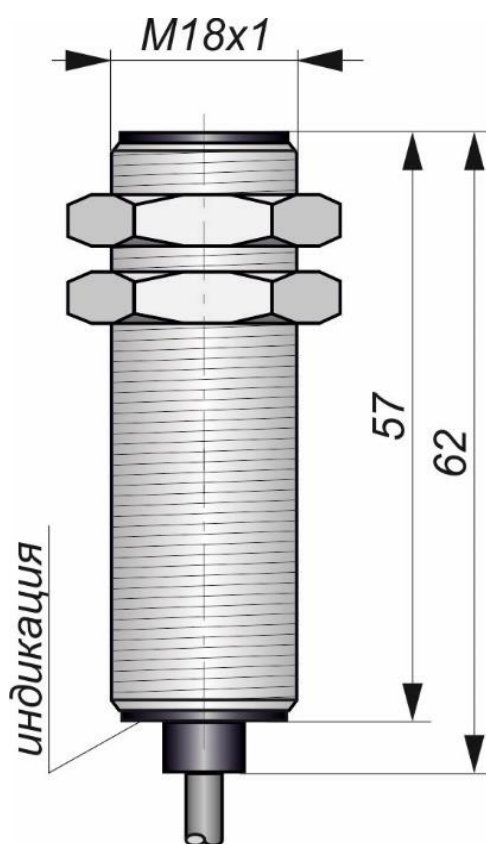
Габаритный чертеж
